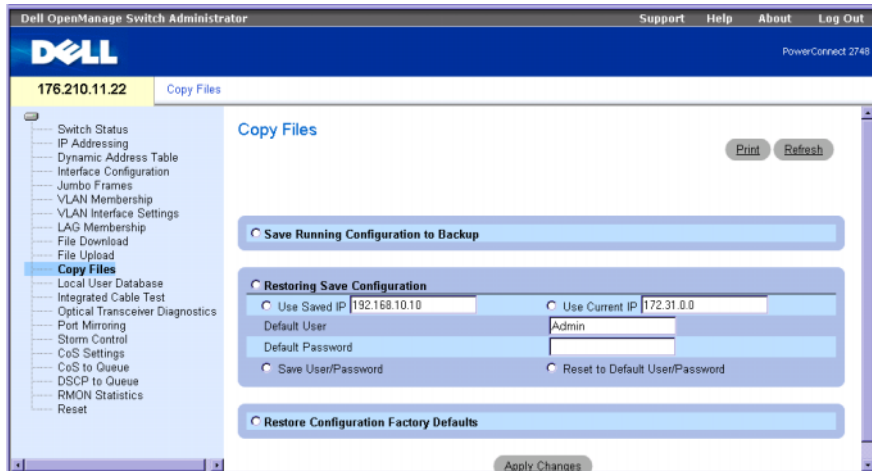
그림 6-11. 파일 복사
